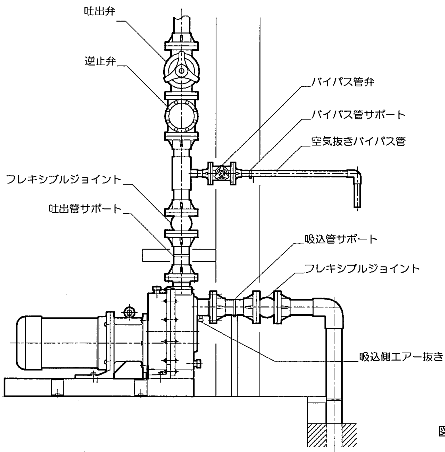
図2 吸込配管
